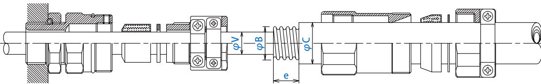
金属管部露出長 e寸法表
