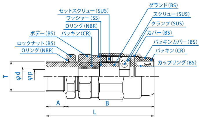
型式：寸法一覧表
