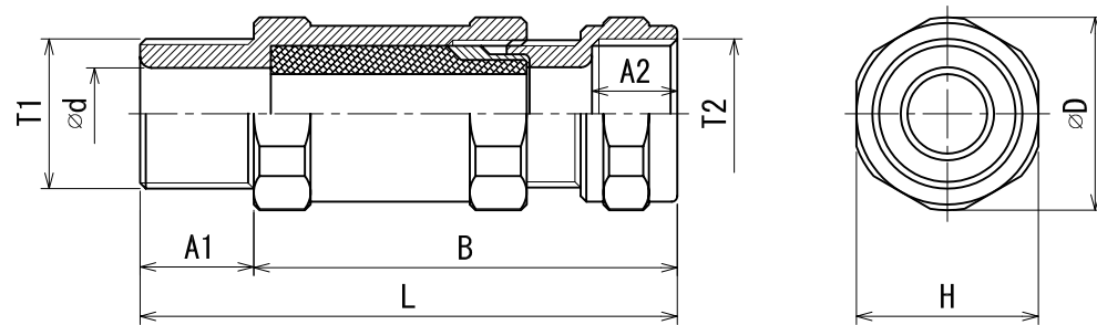
型式：寸法一覧表
