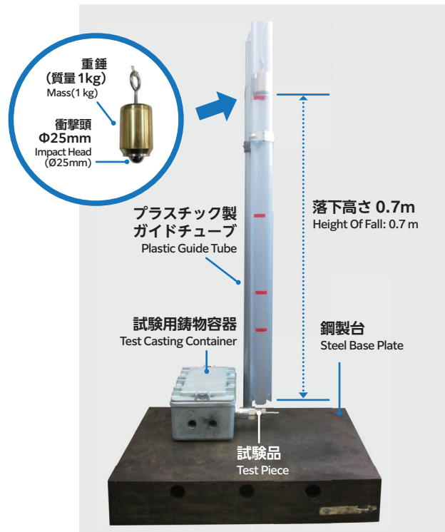
衝撃試験装置 外観 Impact Test Apparatus - External View
