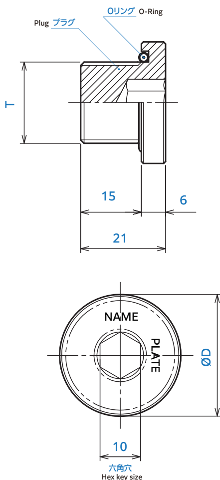
型式：寸法一覧表 Type / Dimensional Specification Table
