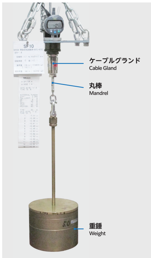
引留機能試験装置 外観 Test Apparatus - External View
