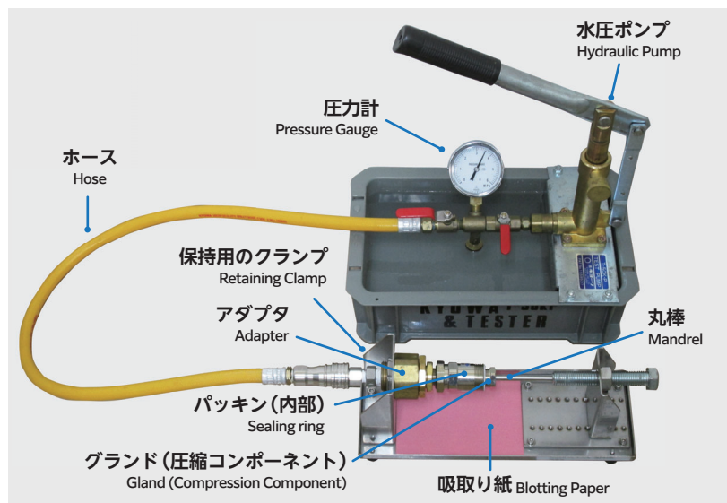
密封性試験の装置 Sealing Test Apparatus
